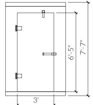
36" WIDE DOOR
