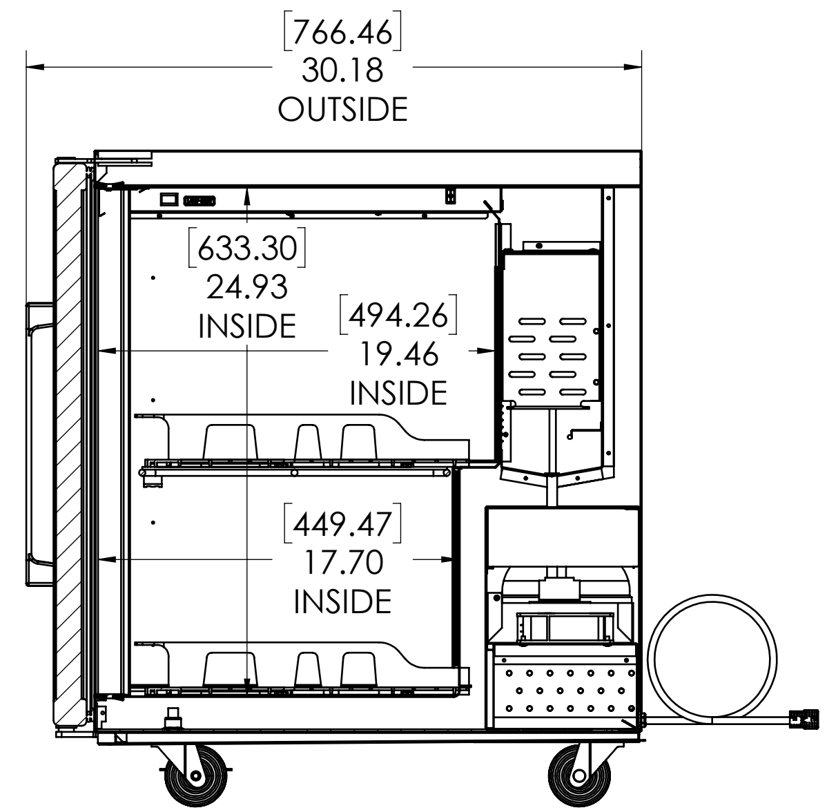
SECTION A-A
