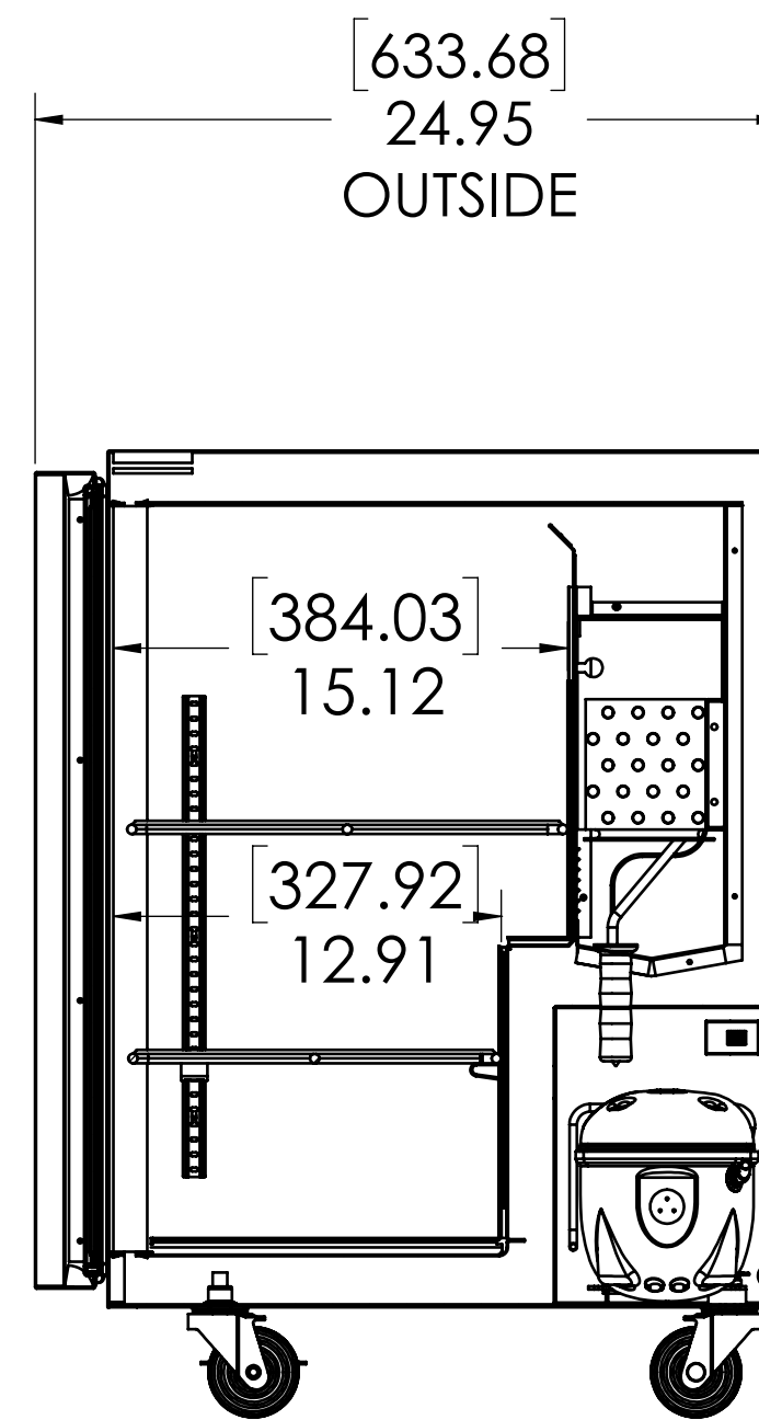
SECTION A-A
