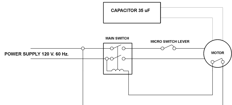
Fig. n°12 - Wiring diagram
