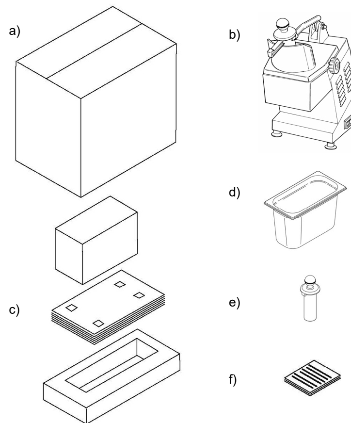
Fig. n°9 - Package description
