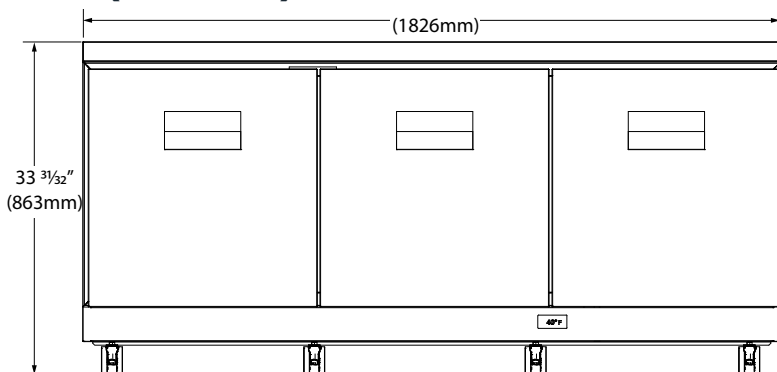
Front (UCFZ372)
