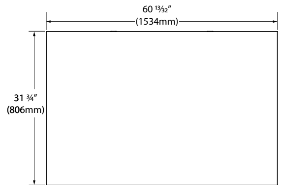
Top (UCFZ360)
