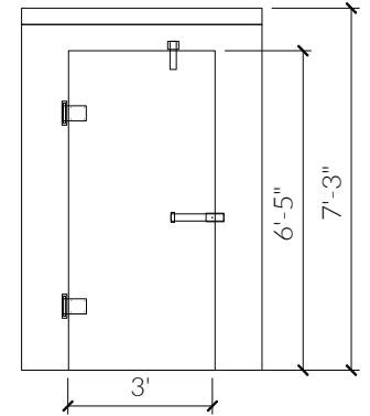
36" WIDE DOOR
