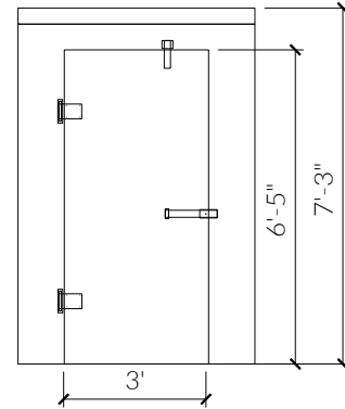
36" WIDE DOOR
